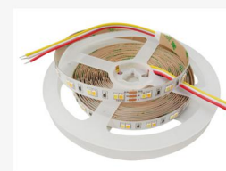
型号: 24V-120A 名称: 24V 裸板双色温灯带 (120灯) 规格: 24V 2835 120LED/M 13W 裸板 两端出3线
