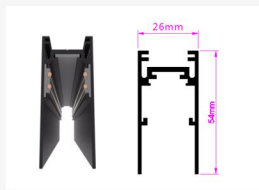
型号: G006-1 名称: 20明装/吊装轨道, 黑色 规格: 宽26mm*高54mm, 长1m, 2m 可选
