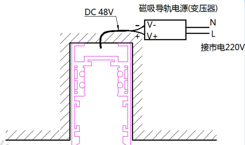
型号: G011-1 名称: 20批灰款轨道, 黑色 规格: 宽26mm*高54mm, 长1m, 2m 可选
