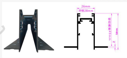
型号: G011-1 名称: 20批灰款轨道, 黑色 规格: 宽26mm*高54mm, 长1m, 2m 可选
