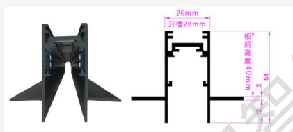
型号: G012-1 名称: 20暗装轨道, 黑色 规格: 宽26mm*高54mm, 长1m, 2m 可选
